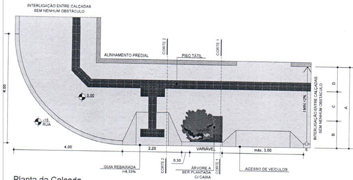
Planta da Calçada Passeio Padrão
